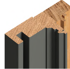
Rolluikgeleider
