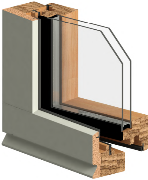
Opendraaiende vleugel
